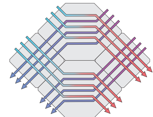
■ Принцип действия комби-теплообменника
